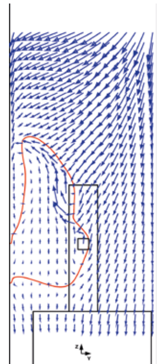
↑ FIGURE 6 Vitesses d'air dans un plan vertical proche de la source de pollution, pour une ventilation descendante et une puissance thermique de la source de 9 900 W.
